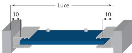
Soluzione 3 = Rilevamento misure in larghezza con telaio a sporgere
