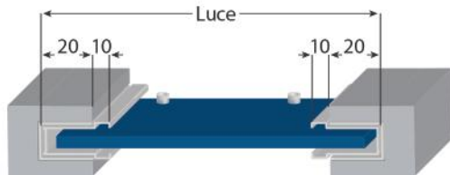
Soluzione 1 = Rilevamento misure in larghezza con inserimento di guide in alluminio per sostituzione
